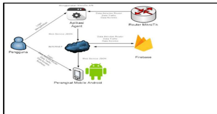
Gambar 4 (a). Arsitektur Sistem pada Aplikasi Monitoring Jaringan Berbasis Android
