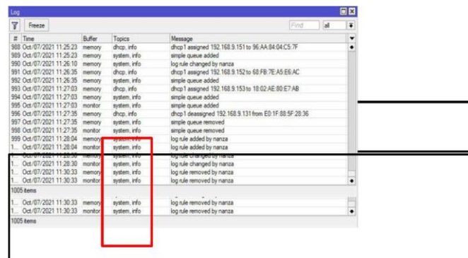
Gambar 4. Pengkondisian Data Log dengan Log Action “monitor”
